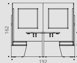
Cabine assise Duo avec bancs vue de face
