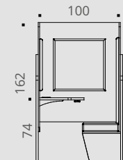
Cabine assise avec banc tablette à gauche vue de face
