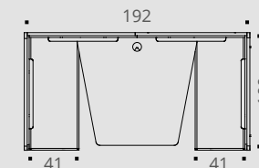
Cabine assise Duo avec bancs vue de dessus
